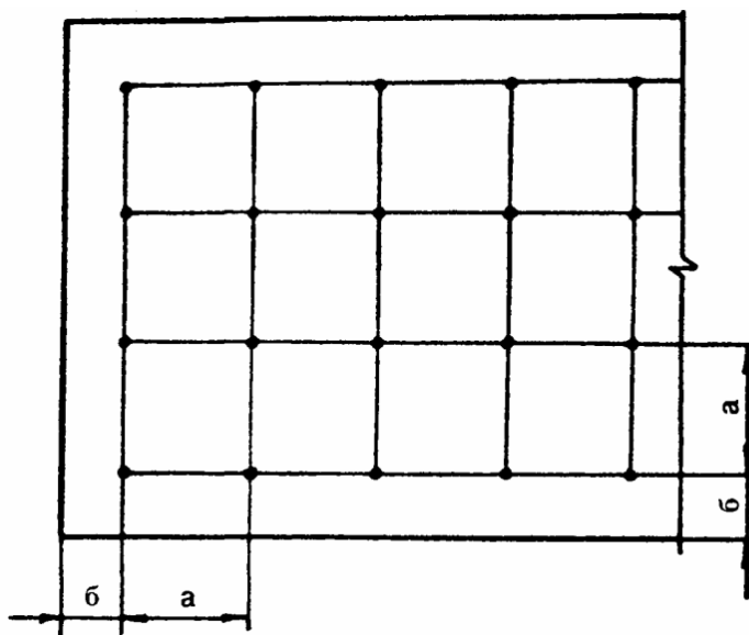
Рисунок 1 – Схема прямоугольного размещения датчиков
