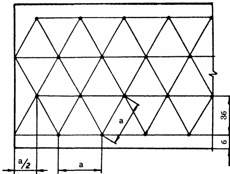
Рисунок 2 – Схема треугольного размещения датчиков
